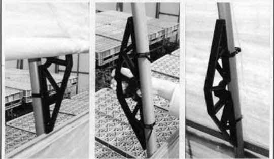
ビニベット上部に「換気名人」を設置します。 ハウス密閉時には「換気名人」をハウス内側へ回し、ハウスを密閉します。
