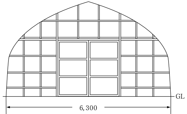
C-38ハウス 間口6.3m (3.5間)
